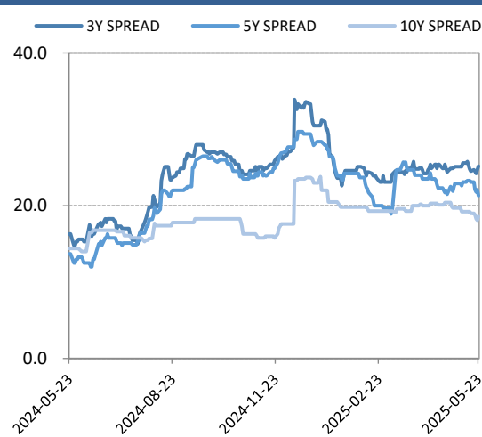
그림4. 특수채AAA SPREAD추이
